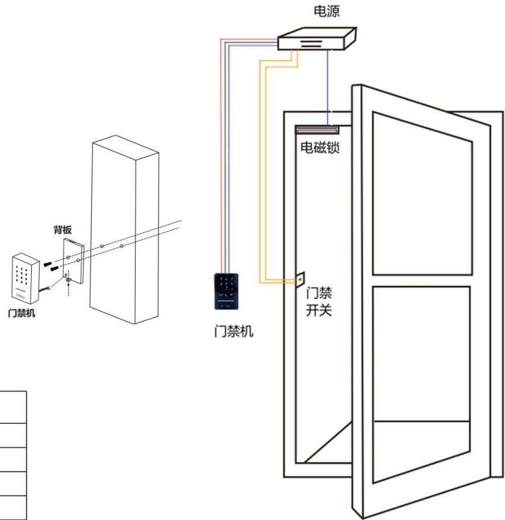
安装示意图
